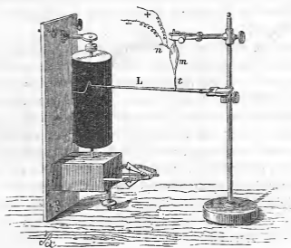
Fig. 2. — Description théorique du myographe.
